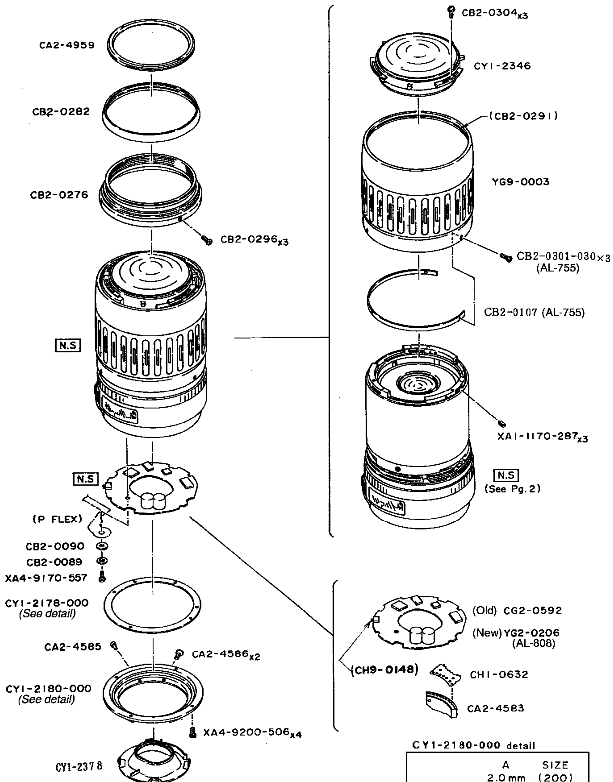
CY1-2178-000 detail
